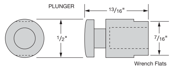
Wrench Flats
